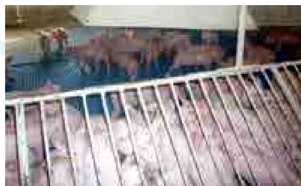
Foto 2 – Leitões aquecidos com resistência elétrica suspensa
