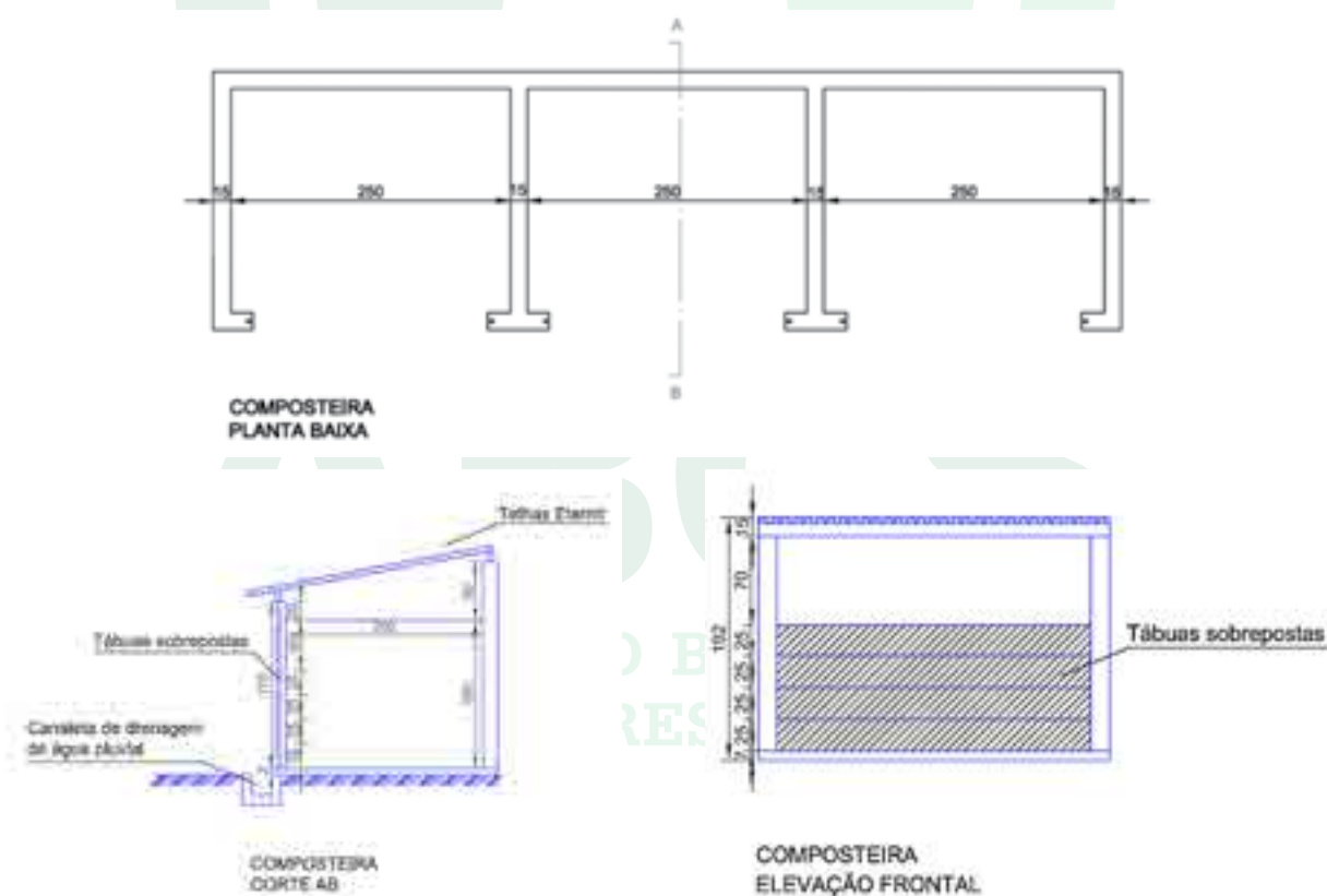
Figura 2 - Planta baixa de um conjunto de células de uma composteira com dimensões de 7,95m x 2,00m, com corte AB, perfil lateral e elevação frontal
