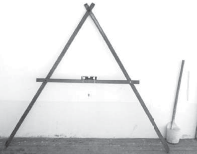
Aparato "A" con plomada y encalador.
